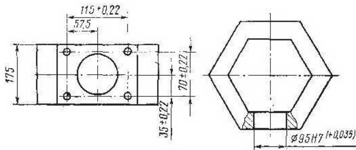
Револьверная головка
