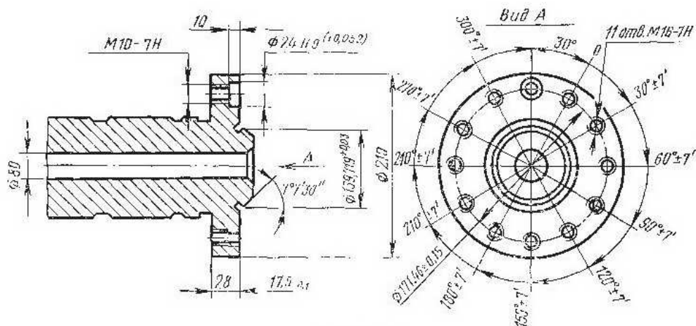
Шпиндель
