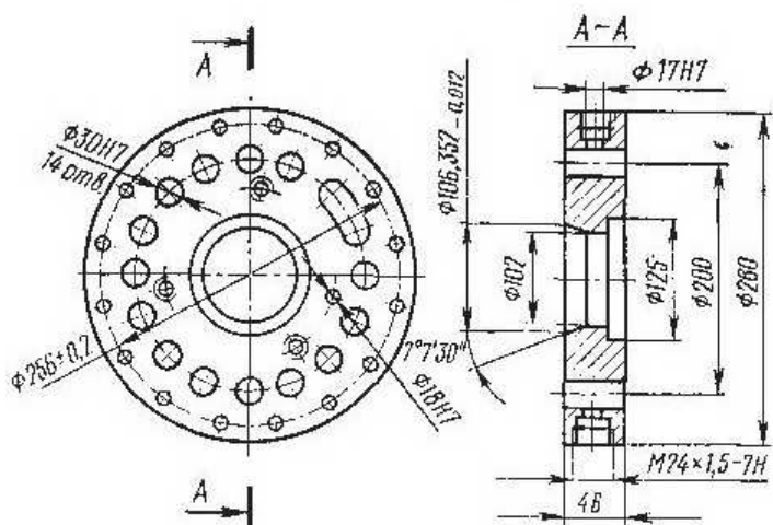
Эскиз револьверной головки
