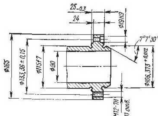
Эскиз конца шпинделя
