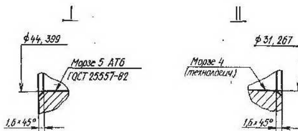
Шпиндель задней бабки
