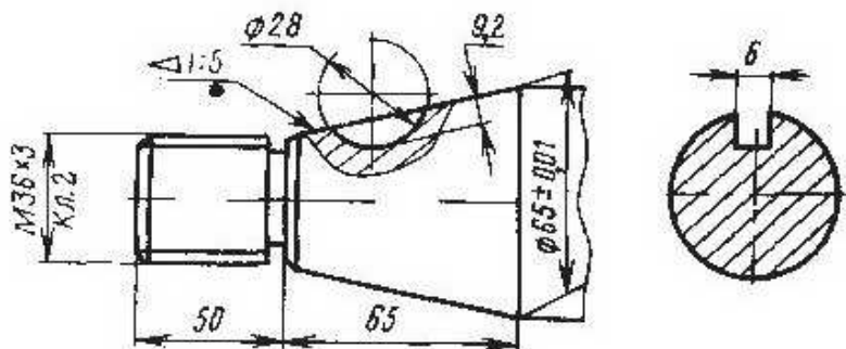
Шпиндель шлифовального круга
