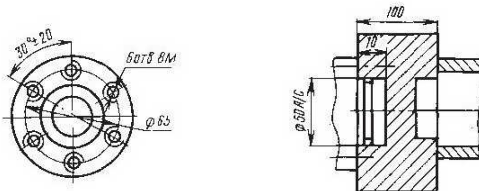
Крепление магнитного патрона
