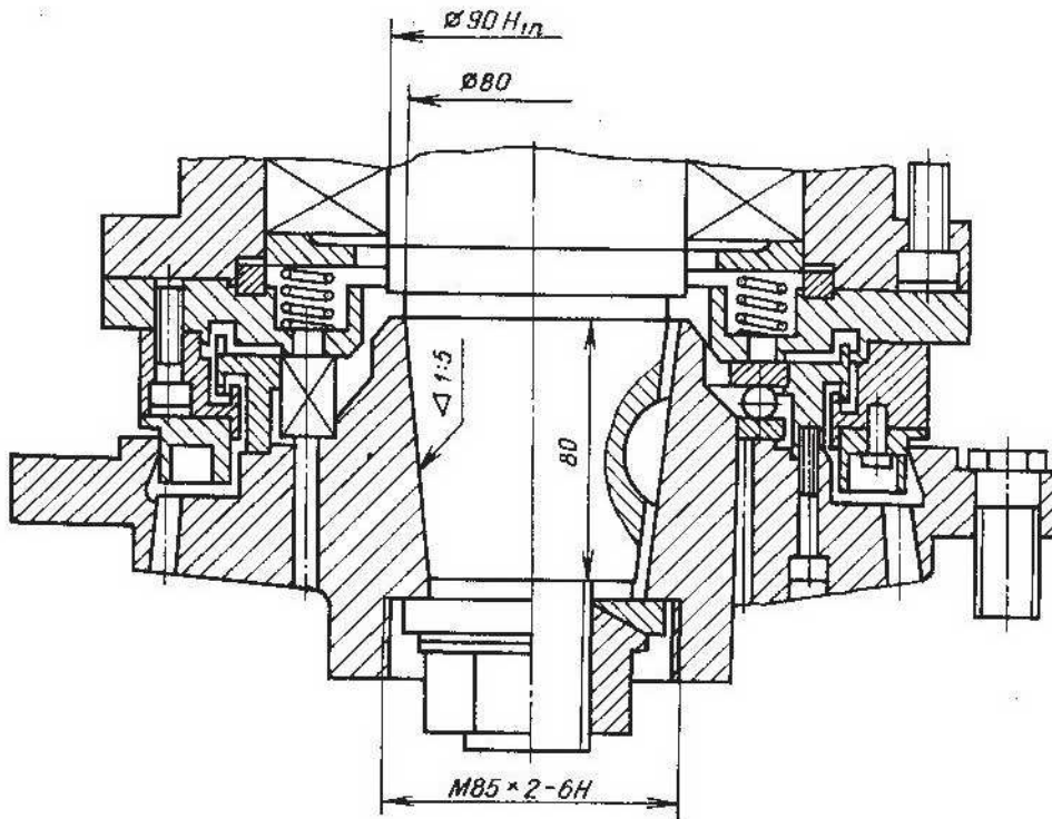
Шпиндель
