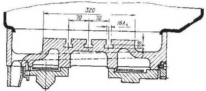
Стол
