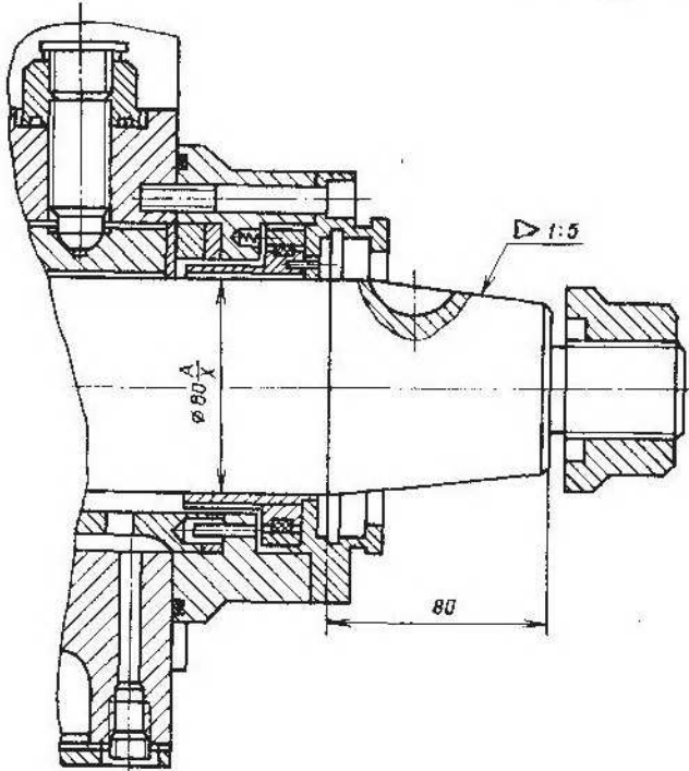
Шпиндель
