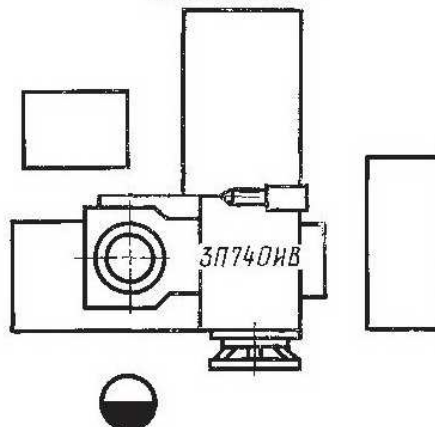
ГАБАРИТНЫЙ ПЛАН Масштаб 1:50
