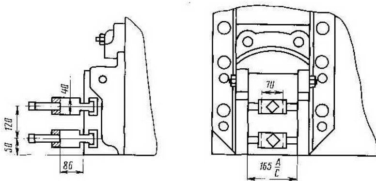
Резцная головка
