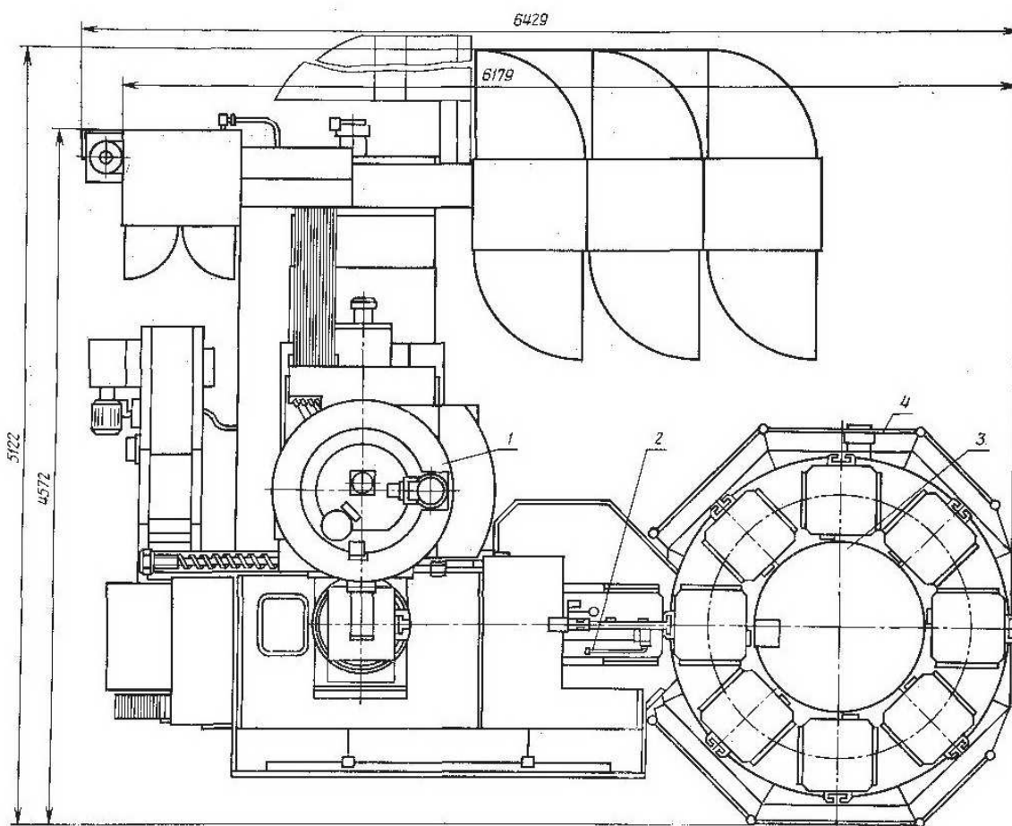
1 — базовый станок; 2 — устройство автоматической смены столов-спутников; 3 — многеместный накопитель; 4 — ограждение
